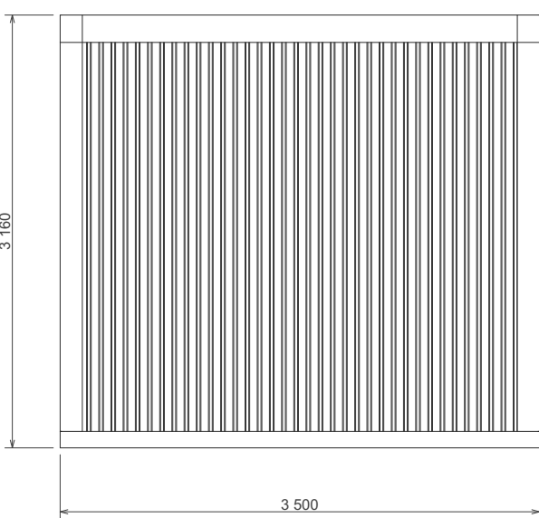
Ansicht Ost
