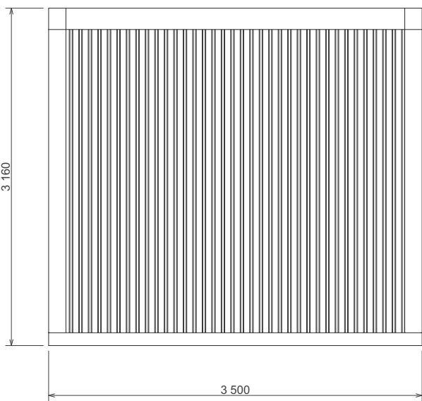
Ansicht Ost
